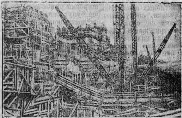
НА СНИМКЕ: Вид на силовую станцию Свирьстрой со стороны верхнего б'ефа
